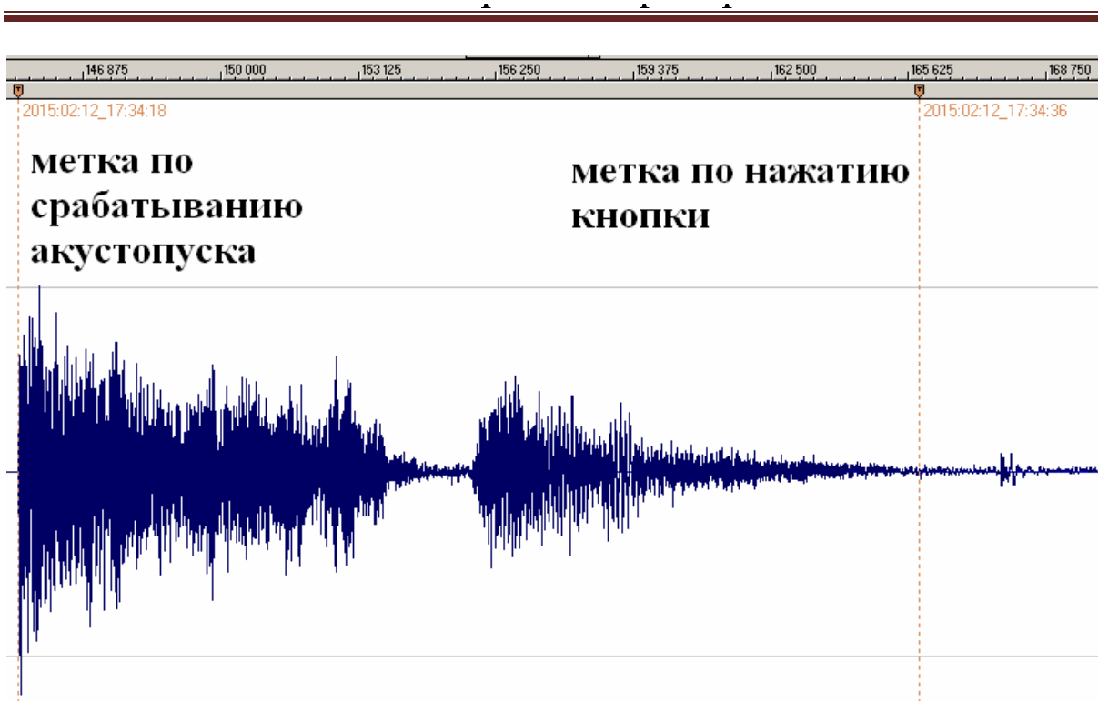
Рис. 8. Пример автоматического распознавания меток программой Sound Forge в аудиофайлах диктофона «Сорока-06». Имя каждой метки соответствует дате и времени ее создания.
