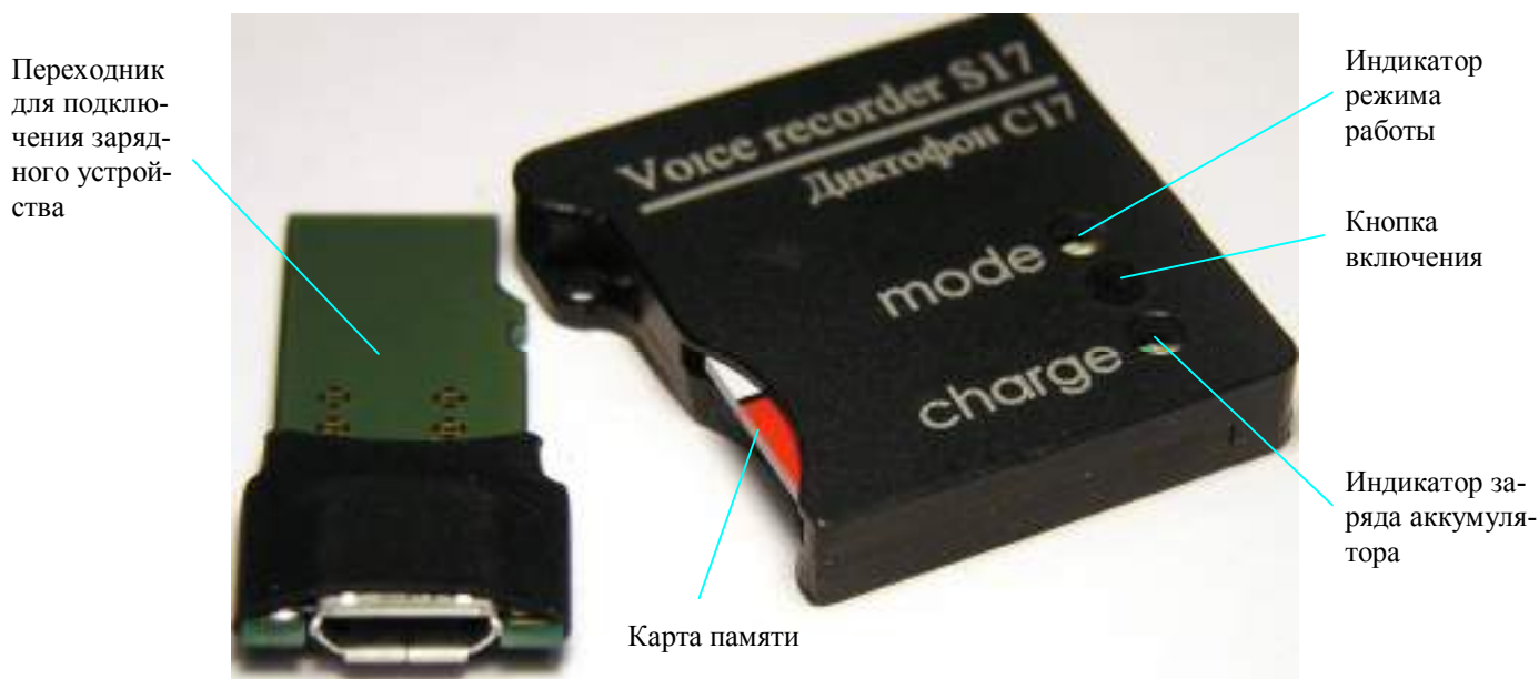
Рис. 2. Внешний вид диктофона «СОРОКА-17».
